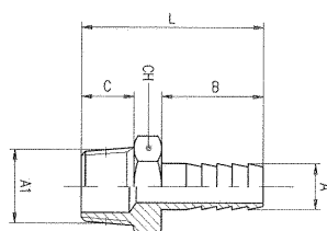
62340 Hadičnick, kuželový závit
